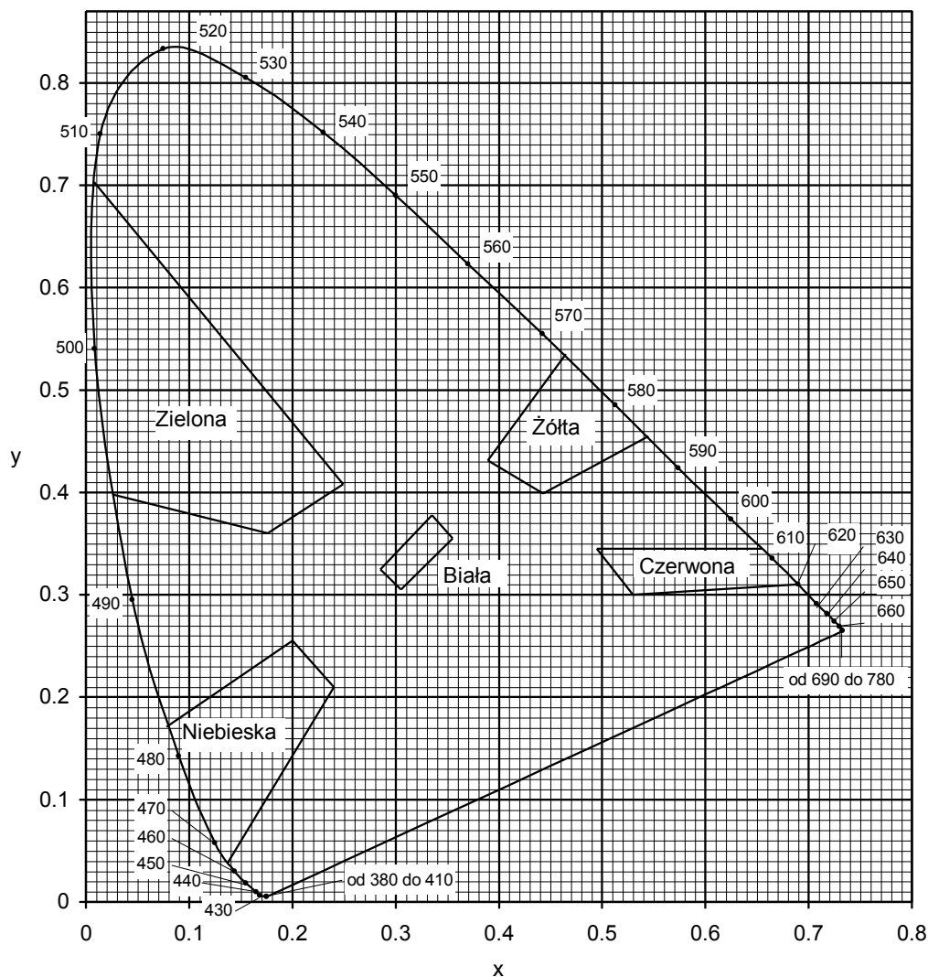
Rysunek 2. Granice barw białej, żółtej, czerwonej, niebieskiej i zielonej oznakowania
