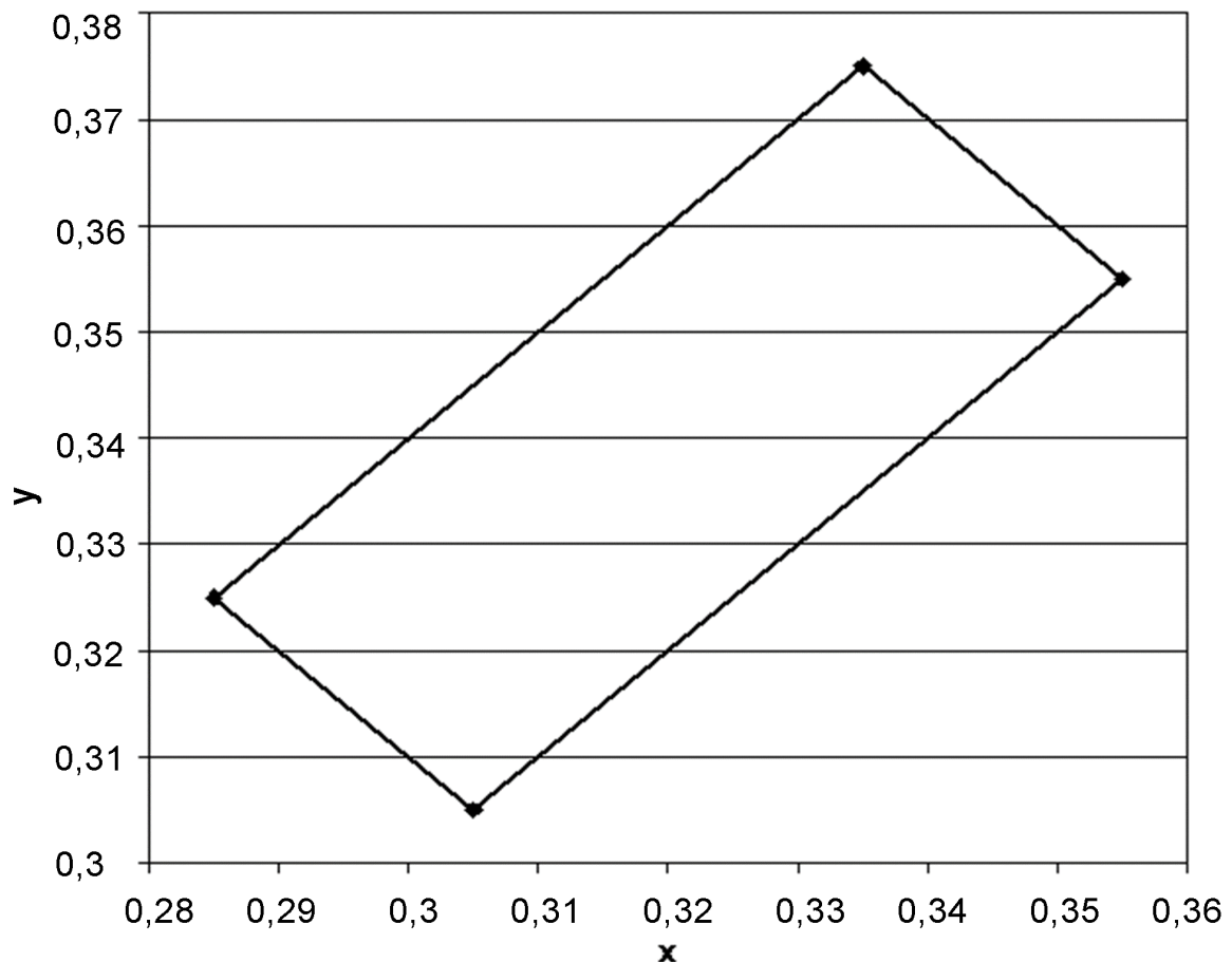
Rysunek 1. Współrzędne chromatyczności x, y dla barwy białej oznakowania
